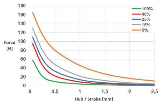
Kraft / Weg-Kennlinie Mit Kühlblech
